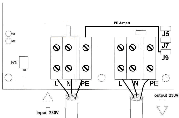
Figure 2 : connexion d'entrée à la terre
